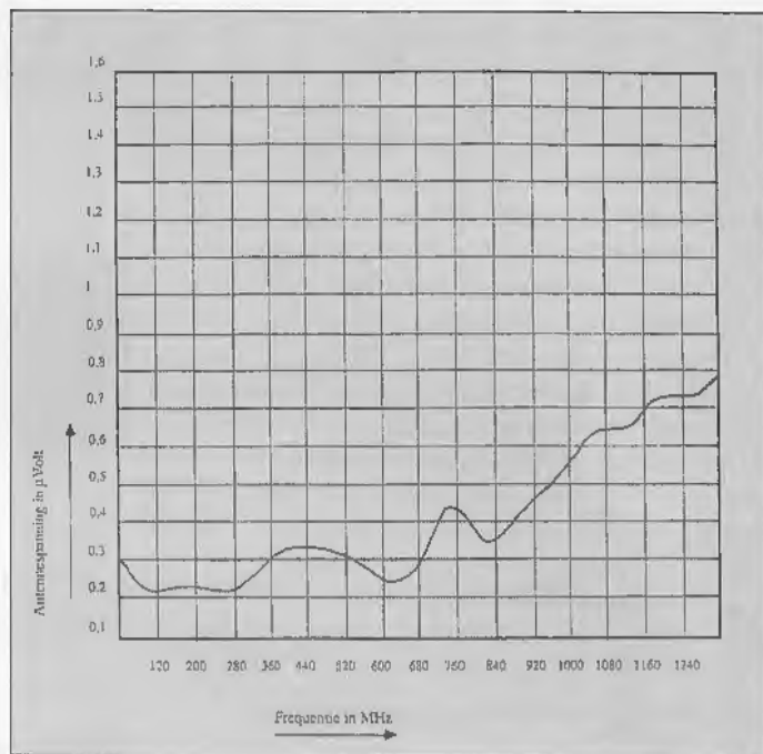
Figuren 1 (links) en 2 (rechts) tonen de gevoeligheid in FM en AM.
